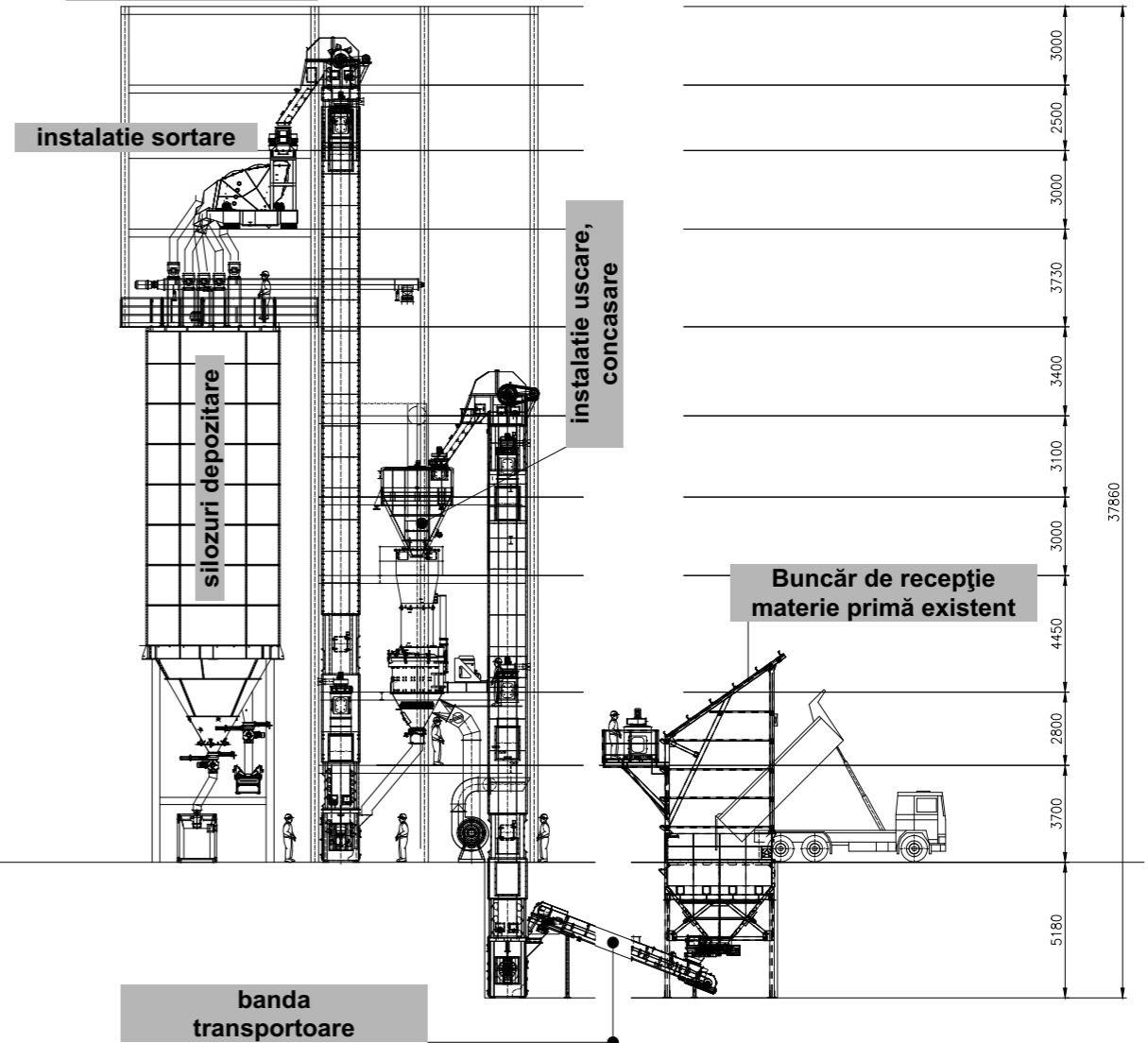
SIMULARE AMPLASARE INSTALATIE PROCESARE NISIP
